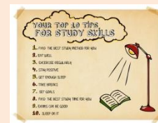
QUEEN : study
